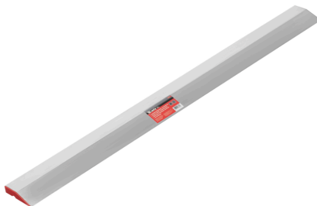
896079 Łata tynkarska aluminiowa trapezowa, 1 żebro wzmacniające, L-1,0 m
